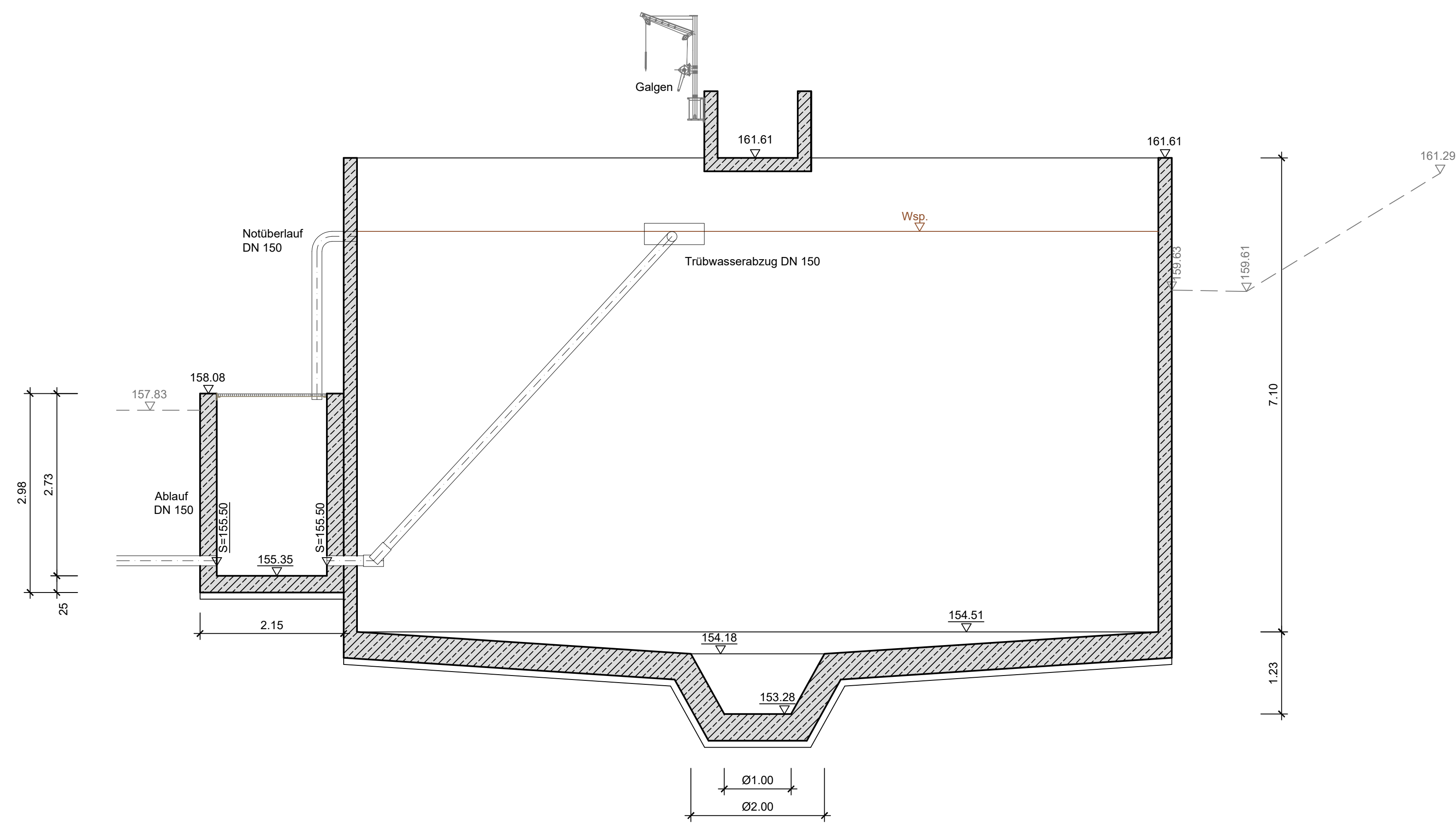
Schnitt A-A
