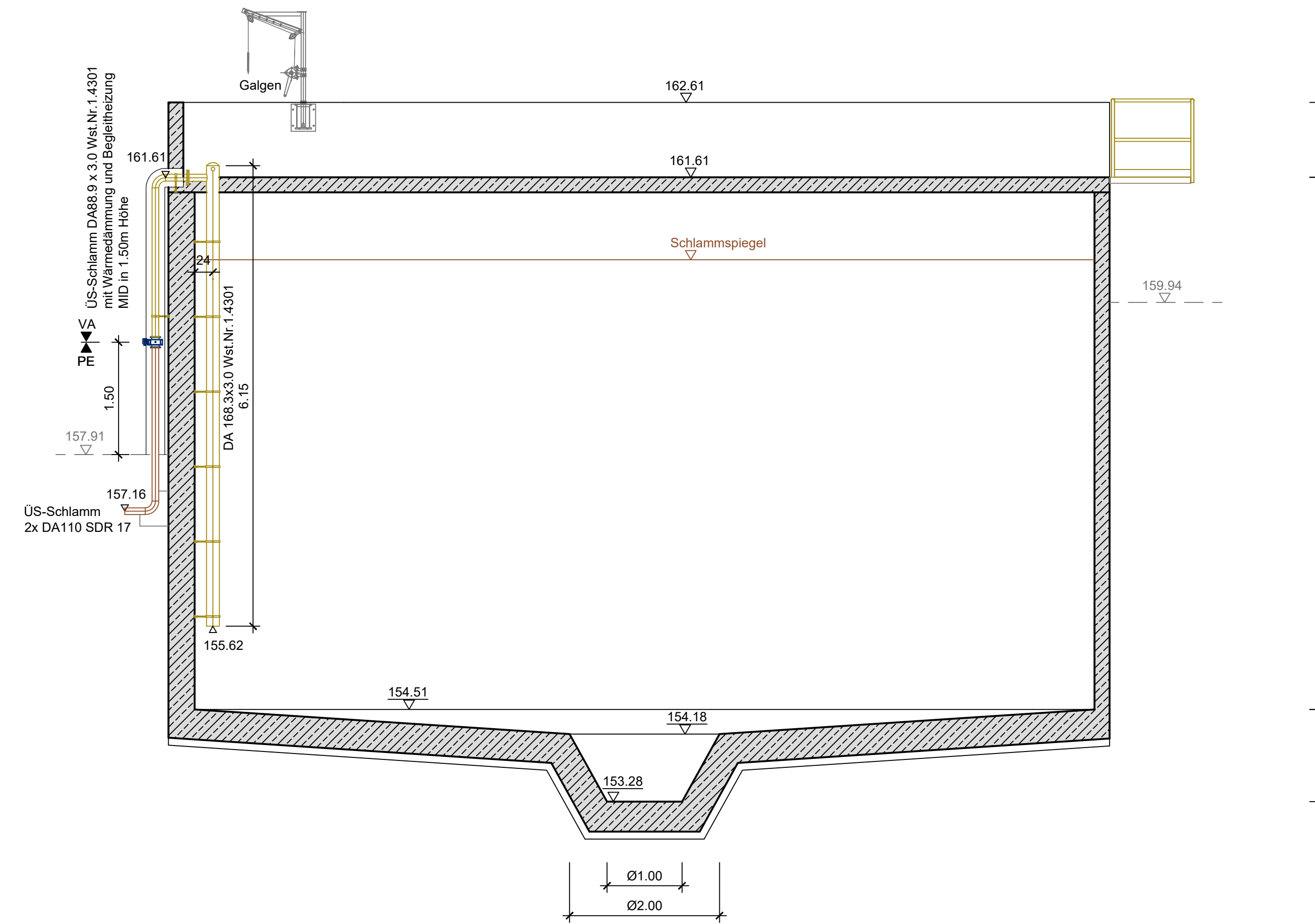
Schnitt B-B
